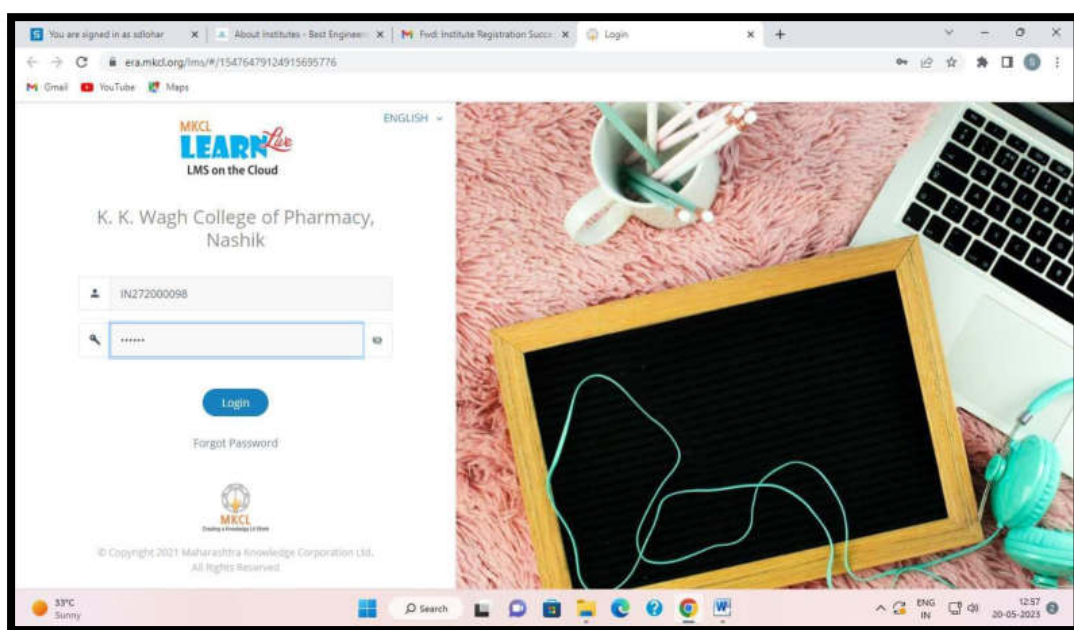
Login Page
